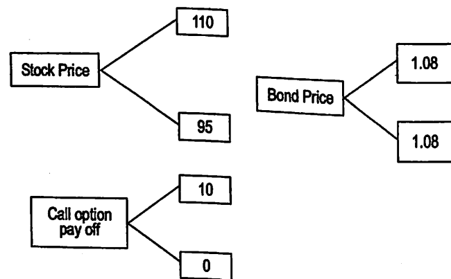
Fig. 9.2 Binomial Model
