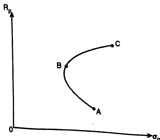
Fig. 8.11 Efficient Frontier
